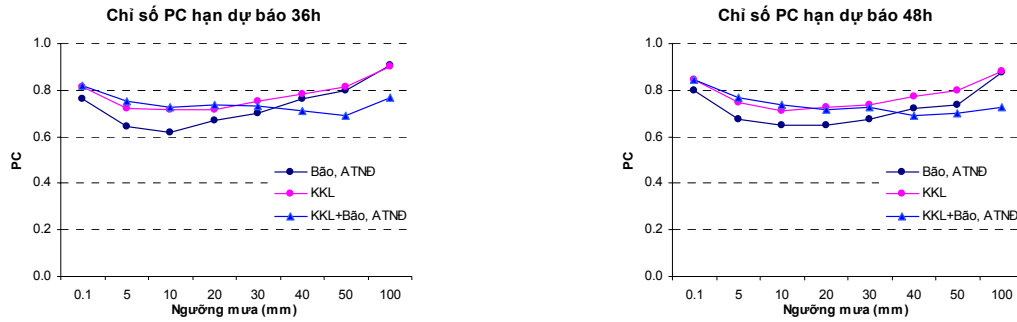
Hình 7. Chỉ số PC tính cho 23 đợt mưa lớn trong các năm 2005-2007
