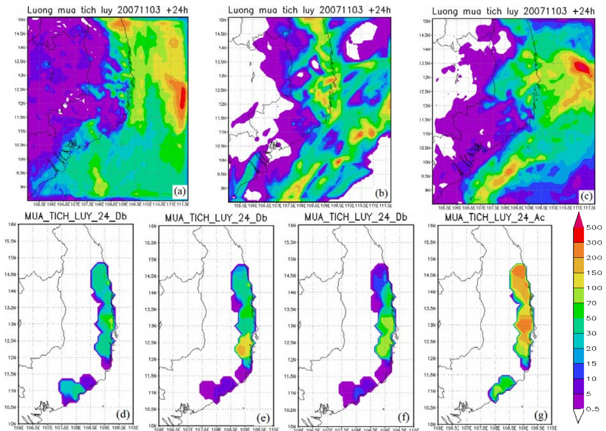
Hình 3. Tương tự hình 2 nhưng là mưa tích lũy 24h
