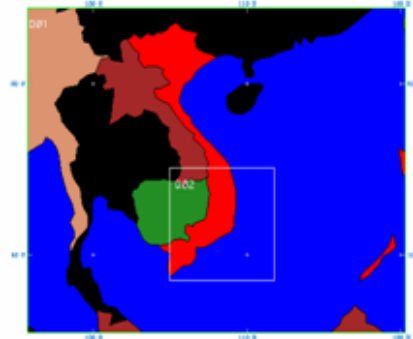
Hình 1. Miền tính của mô hình
