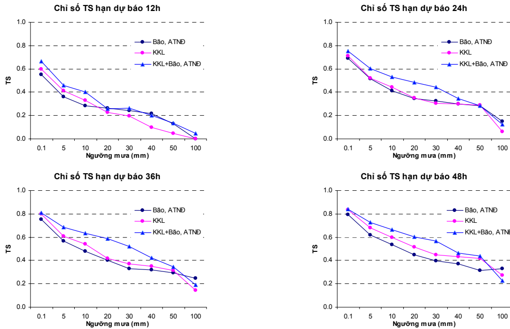
Hình 8. Chỉ số TS tính cho 23 đợt mưa lớn trong các năm 2005-2007
