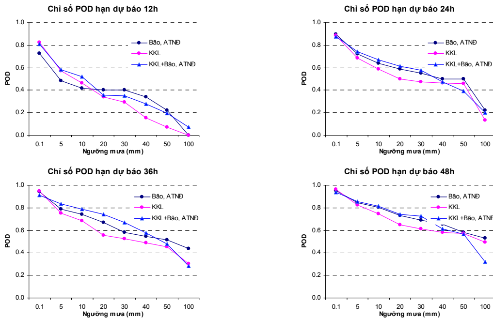
Hình 6. Chi số POD tính cho 23 đợt mưa lớn trong các năm 2005-2007
